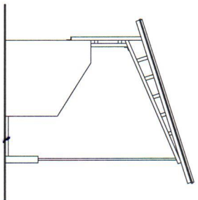
ESTADIO PARA BASEBALL ELEVACION LATERAL IZQUIERDA 1:50
