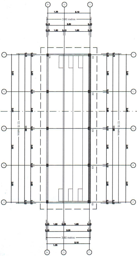
ESTADIO PARA BASEBALL PLANTA ARQ. DIMENSIONADA GRADERIAS 1:50
